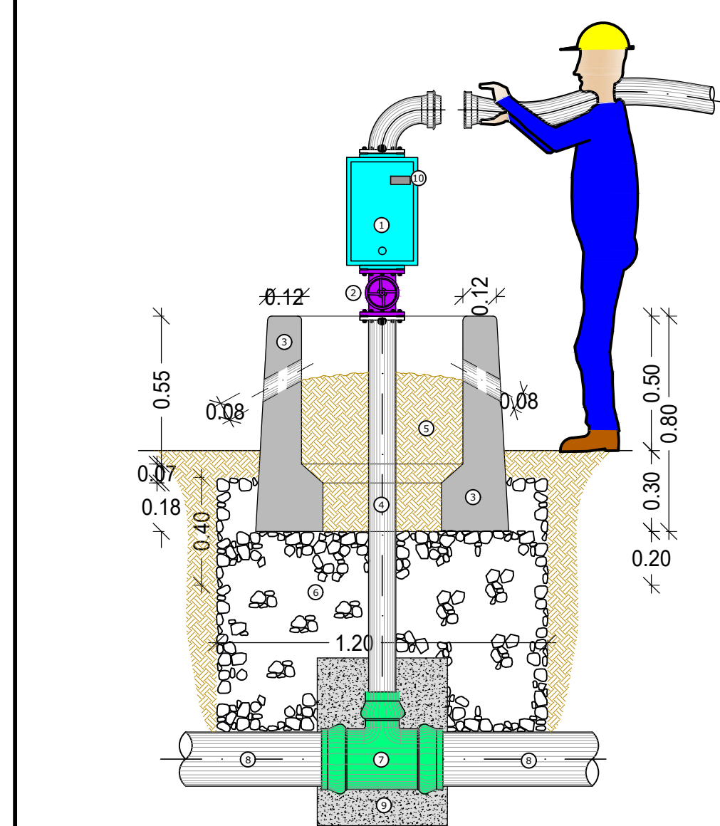
POZZETTO PREFABBRICATO
