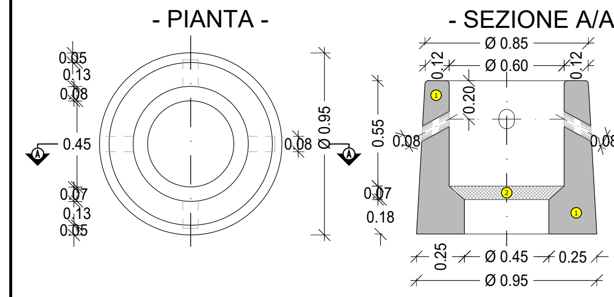
POZZETTO PREFABBRICATO
